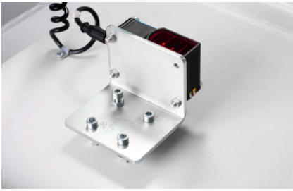
HSM TCS (TorsionControlSystem) para controlar la inclinación de la plancha de prensado
